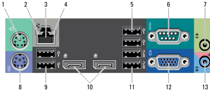
Kuva 2. Takapaneelinäkymä
